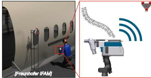
Industrie 4.0 beim semiautomatischen Bohren
