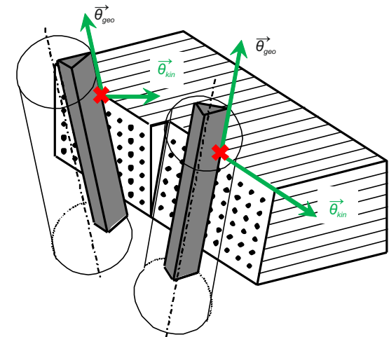
Modellbildung des räumlichen Schneideneingriffs bei UD-CFK
