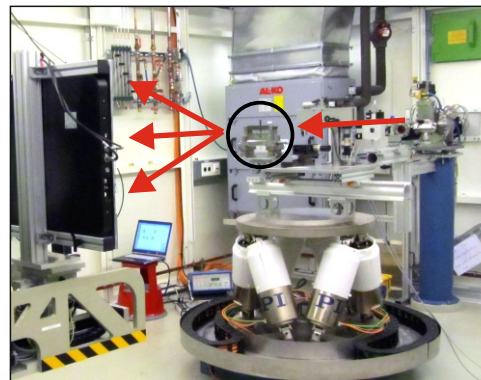
Schneidstoffanalyse mit Synchrotronstrahlung unter thermomechanischer Belastung
