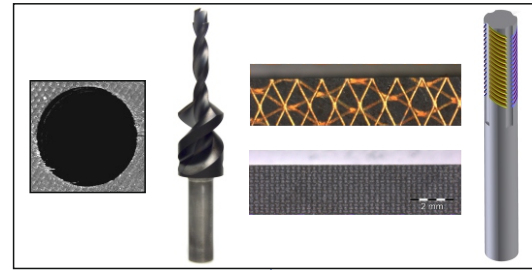
Entwicklung diamantbeschichteter Werkzeuge für CFK
