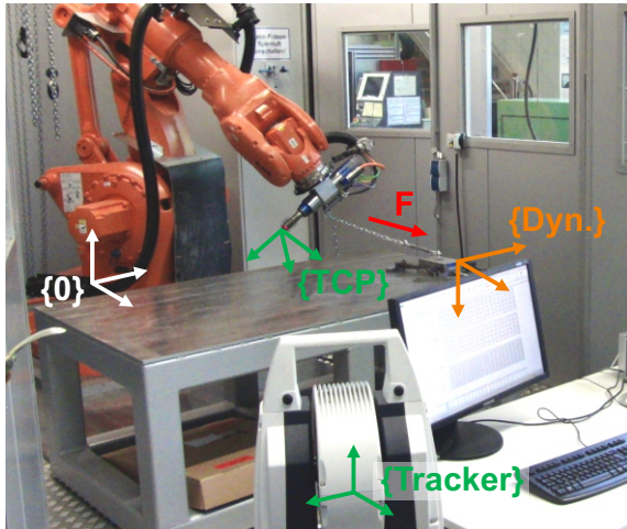
Identifikation der Gelenk- steifigkeiten eines Roboters
