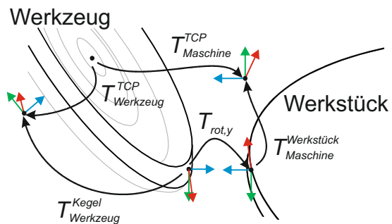
Bahnplanung zum Curved Circular Cutting
