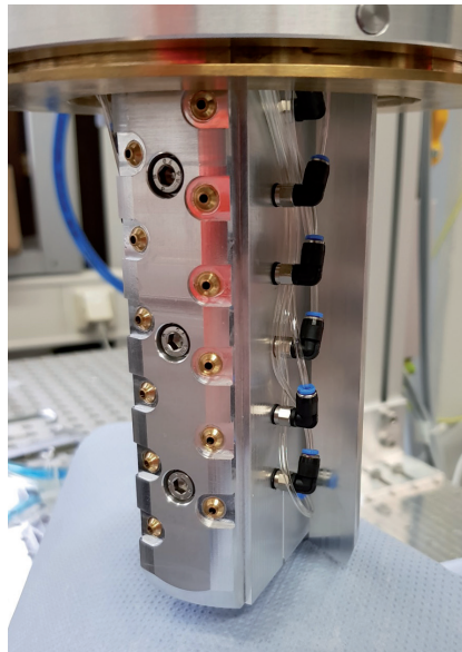
Am Lehrstuhl entwickelte pneumatische Mehrstellenmeseinrichtung für die Inprozess-Messung
