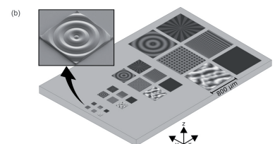
Universalnormal zur Überprüfung der metrologischen Eigenschaften nach ISO 25178-600 von optischen Topografiemessplätzen (hergestellt von Opti-Cal GmbH)
